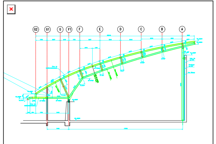
Coupe sur arc du Gymnase
